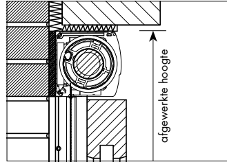
Opbouw , omgekeerde kast bovenop het raam (standaard zonder voorlap)
