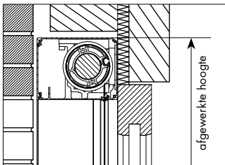
Voorbouw , voor / boven het raam
