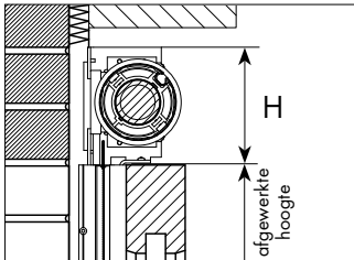
Inbouw , met beugels (zonder kast)
