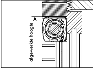
Voorbouw , voor het raam buiten
