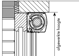
Voorbouw , voor het raam binnen
